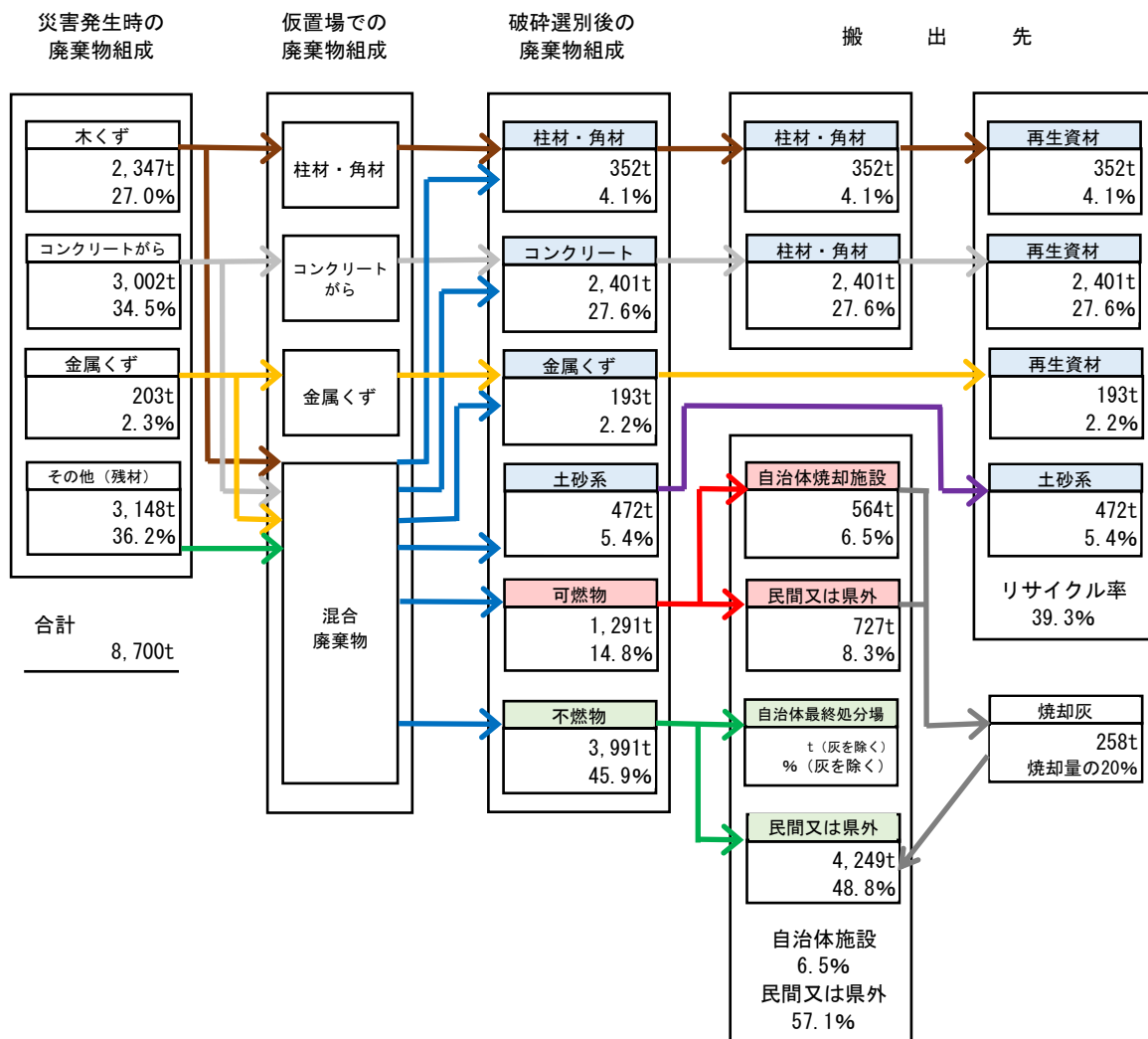
図 1 2 鳥取県西部地震断層の地震における災害廃棄物処理フロー
