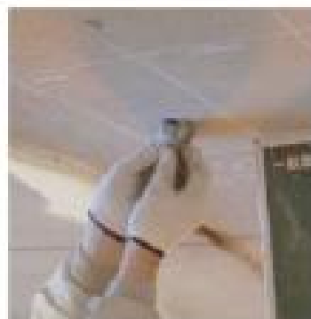
写真 5-7 閉塞状況（無収縮モルタル）
