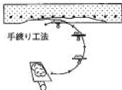
図 6.4 断面修復工概要図
