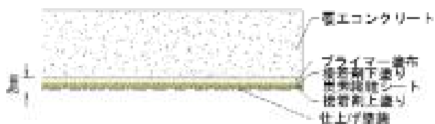
図 6.5 炭素繊維シート工概要図
